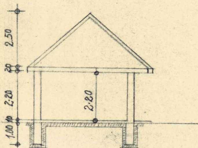
SCHNITT A-B 1:100
