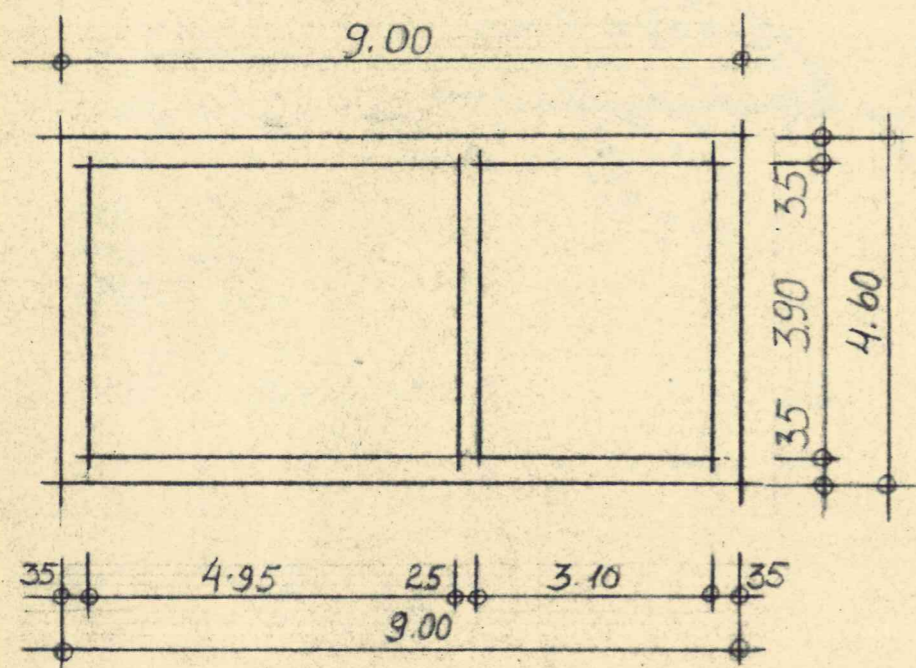
FUNDAMENTE 1:100
