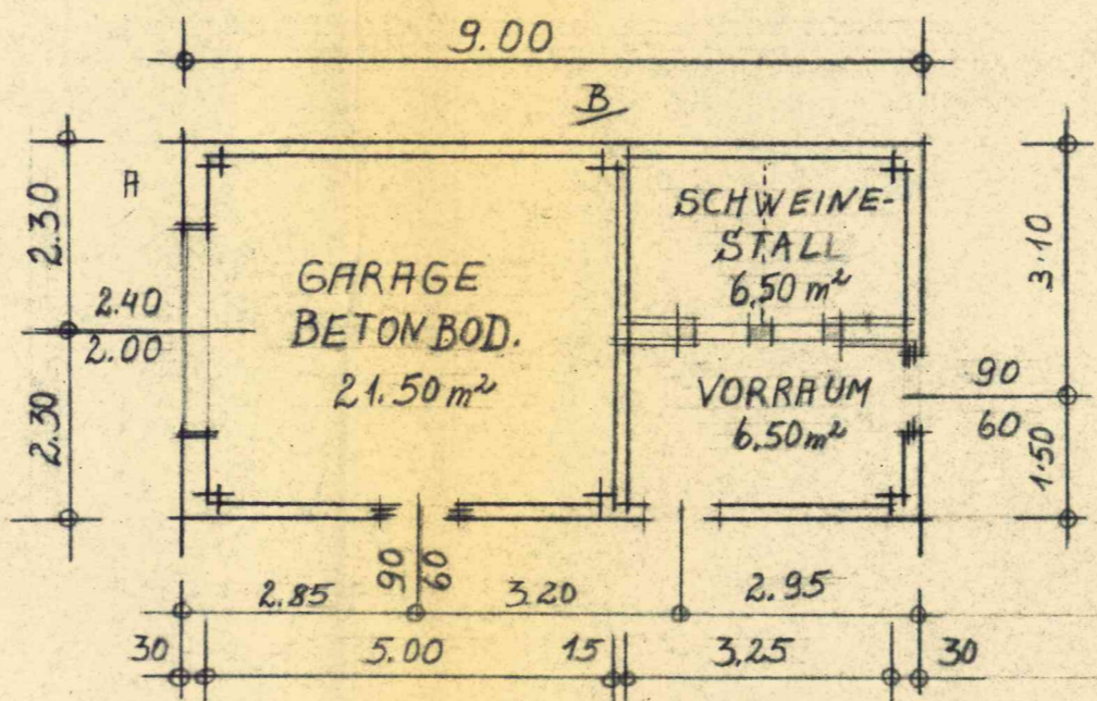
GRUNDRISS 1:100
