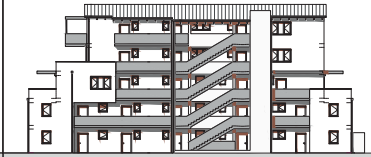
Ansicht Nord
