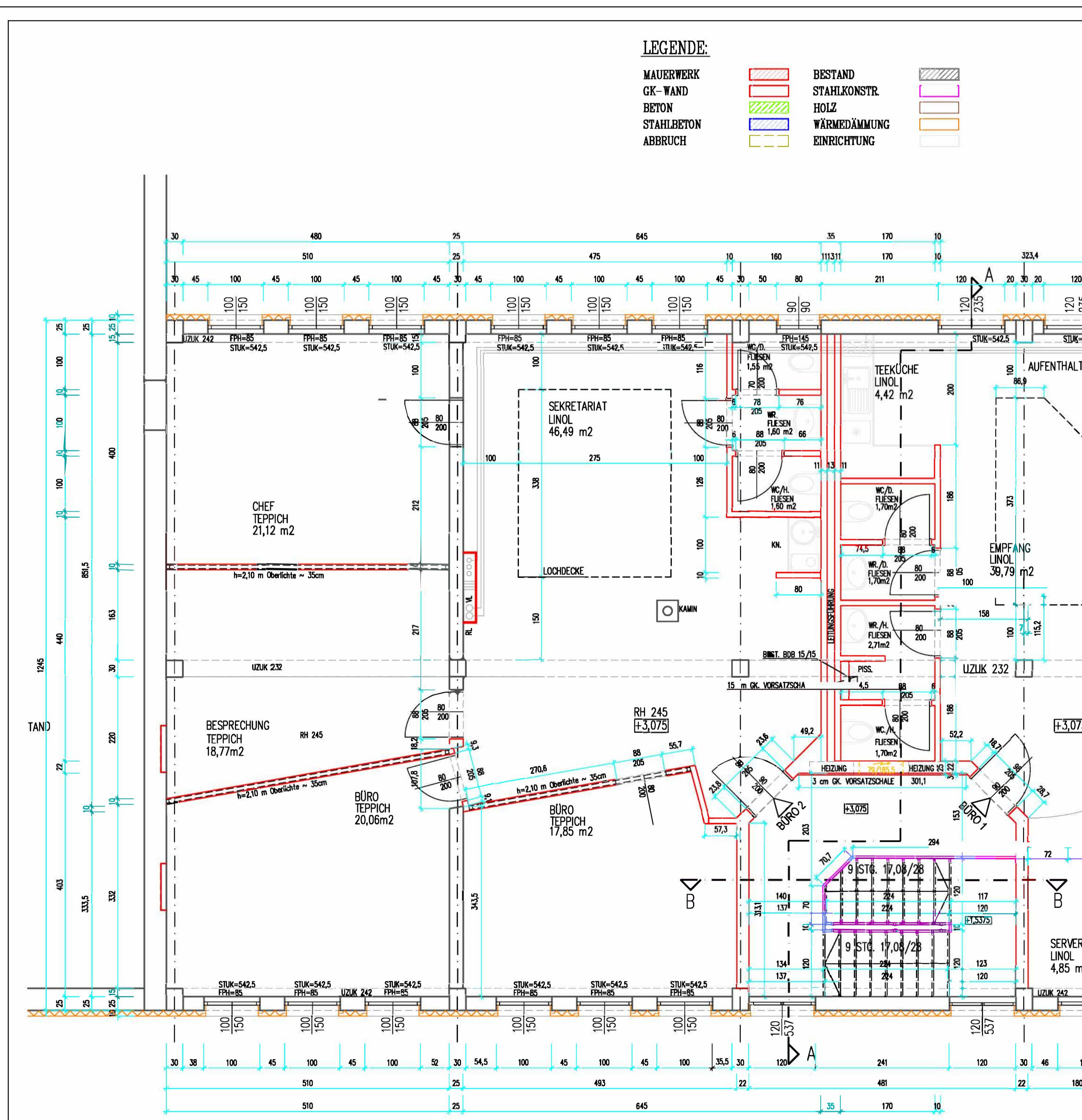
Obergeschoss
