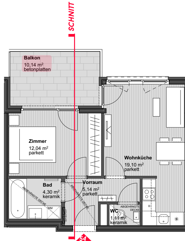
Grundriss | M 1:100
