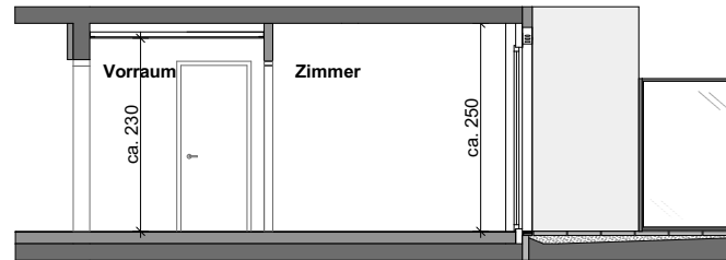
Schnitt | M 1:100
