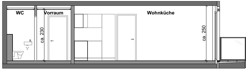
Schnitt | M 1:100
