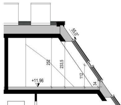
Schnitt 20.B
