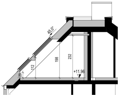
Schnitt 20.A
