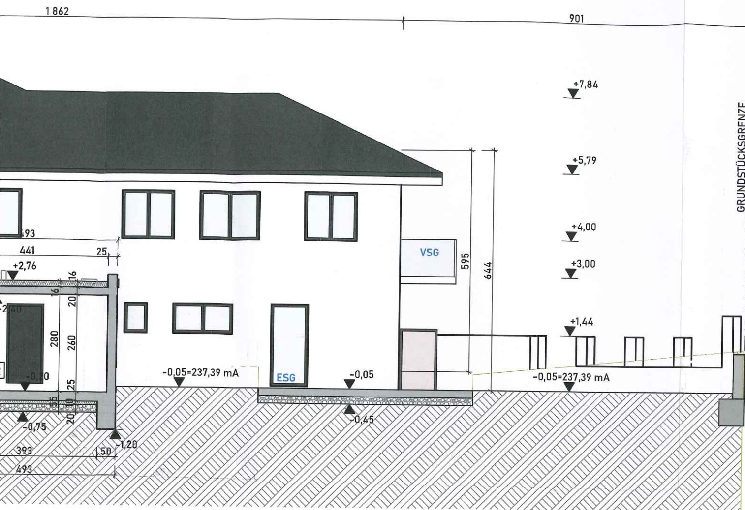
ANSICHT
