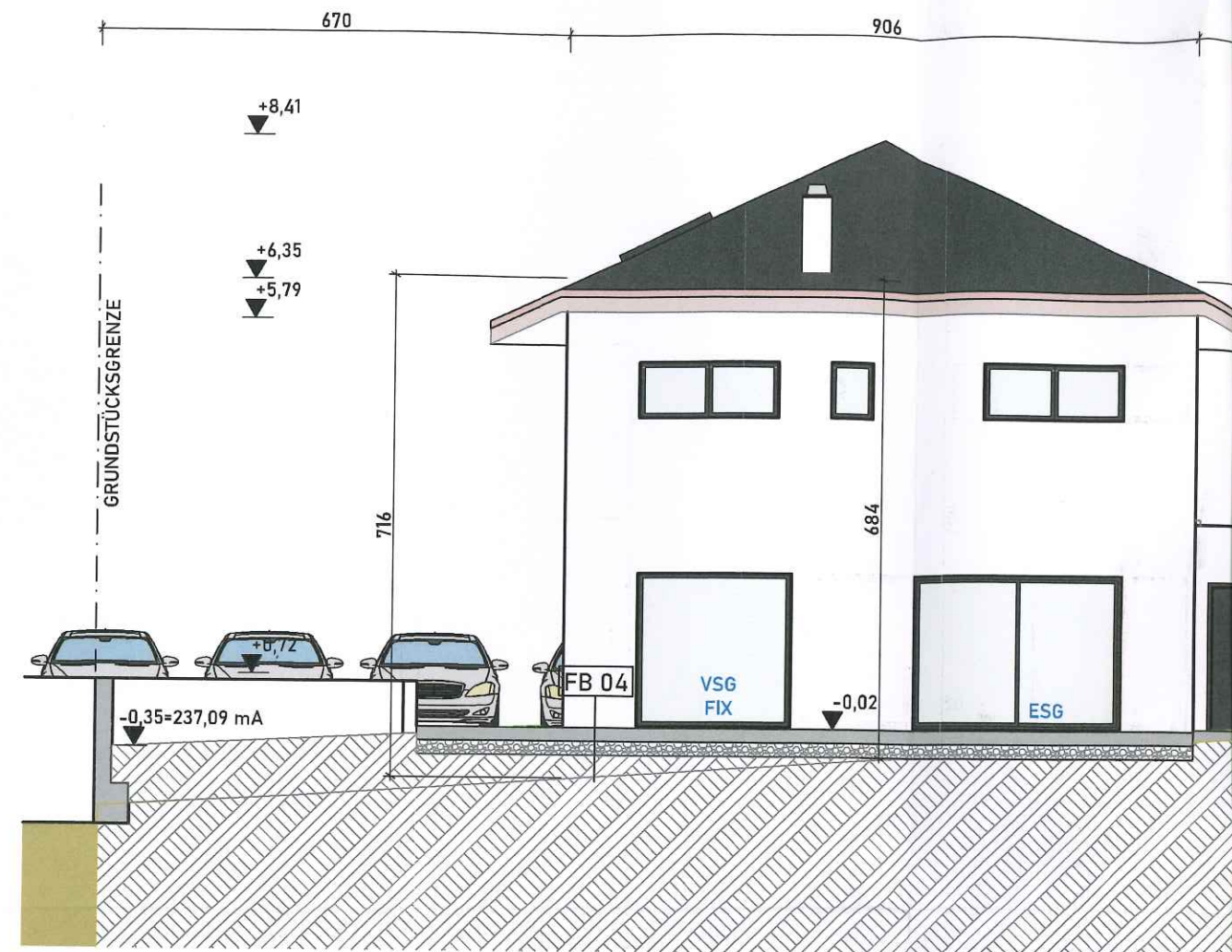
WEST ANSICHT
