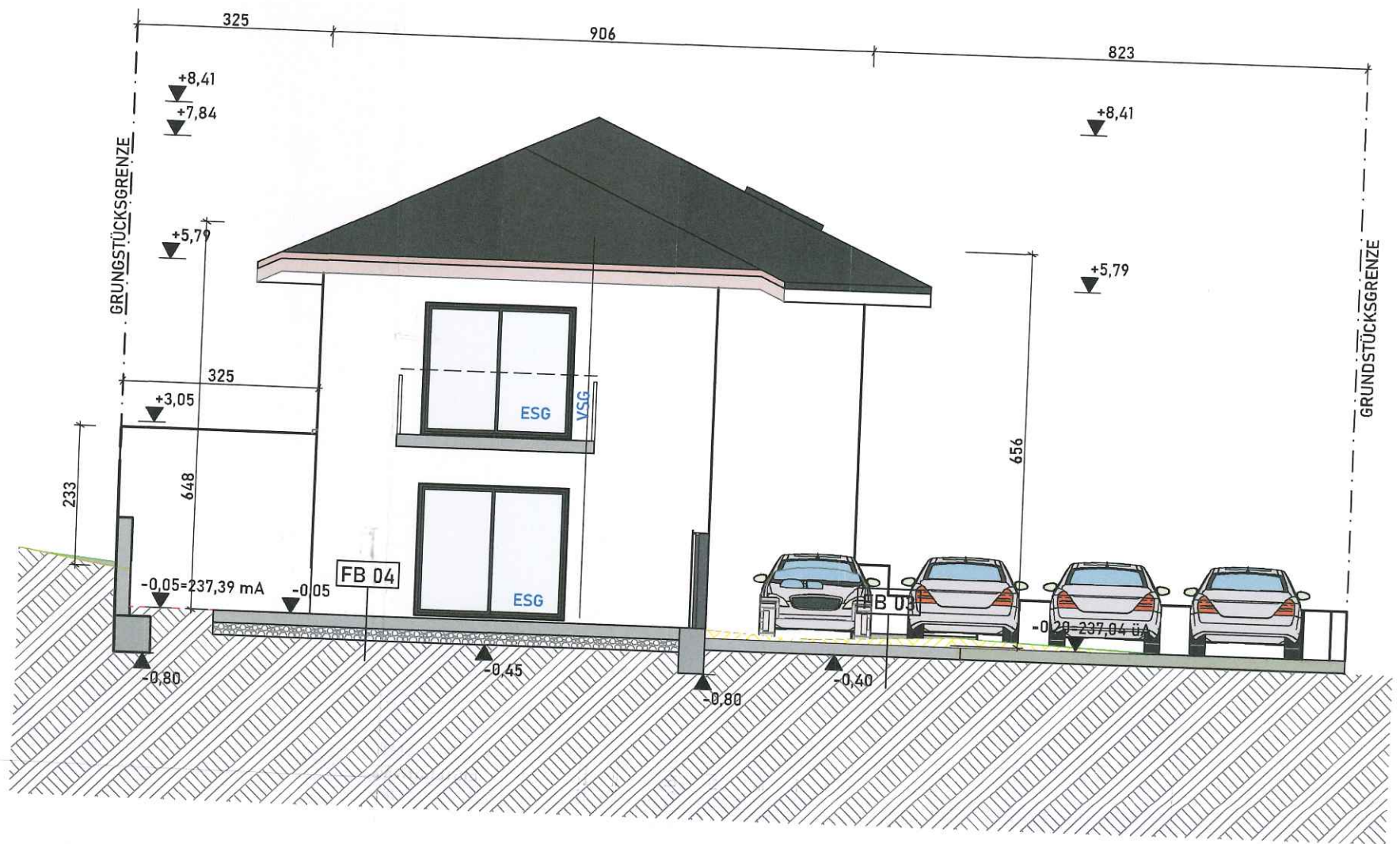
OST ANSICHT
