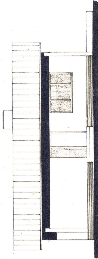
GRUNDRISS
