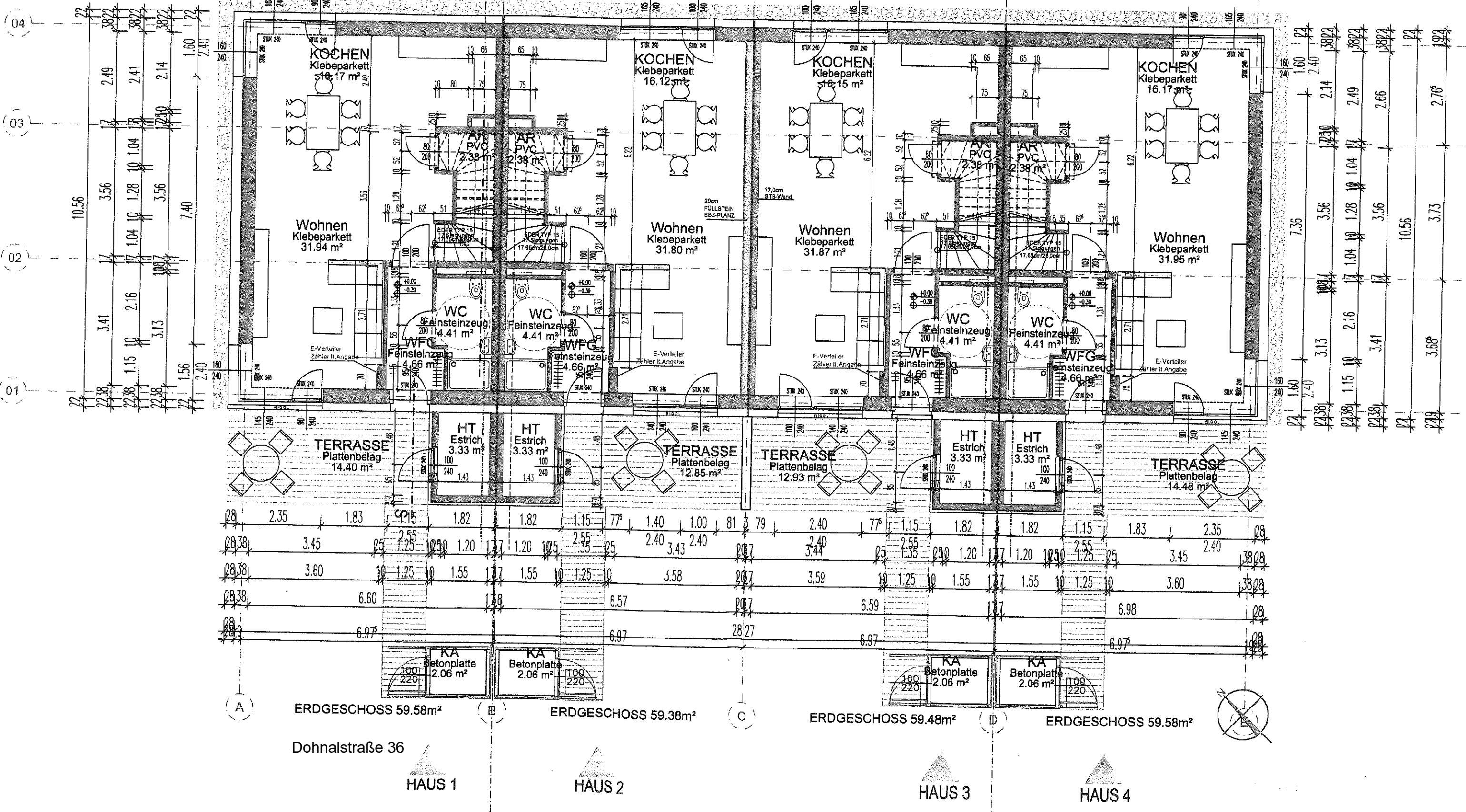
ERDGESCHOSS M 1:100
