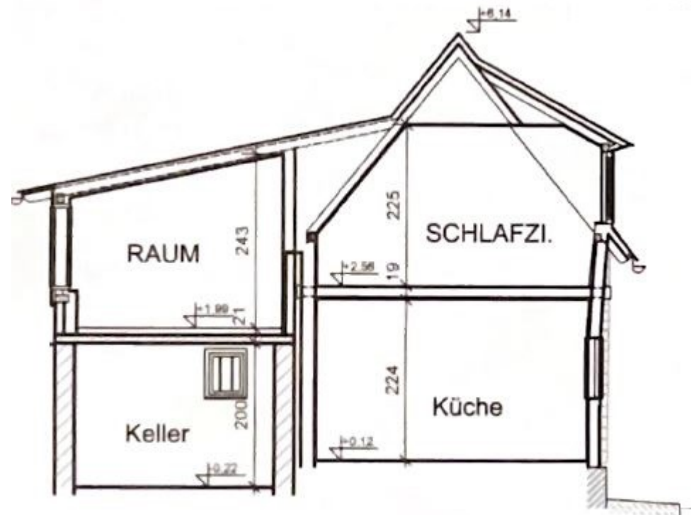
Schnitt A-A
