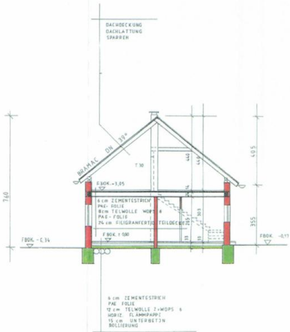
SCHNITT A - B
