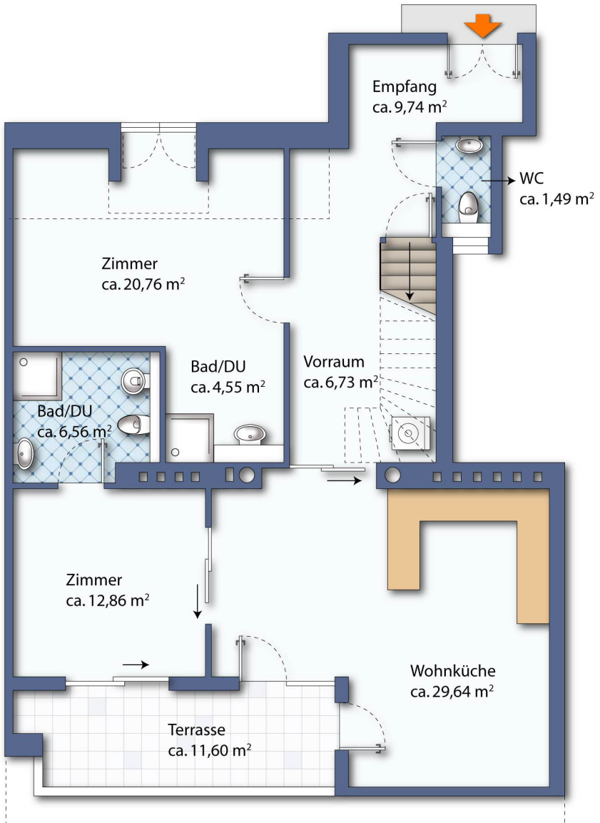
1. Dachgeschoß: Mögliche Grundriss-Variante
