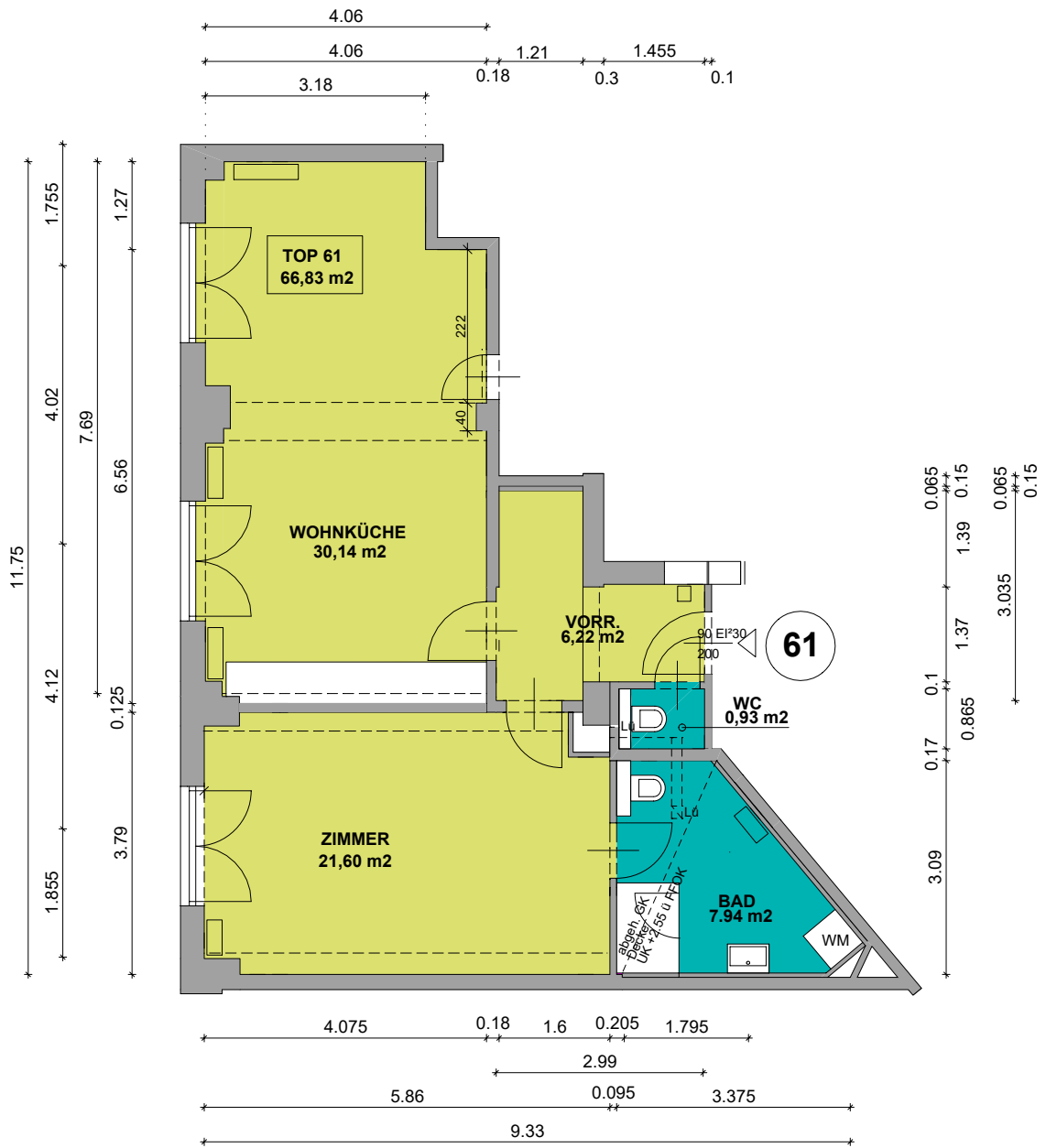
HERRENG. 6-8, STIEGE 1, 10. STOCK, TOP 61, M 1:100
