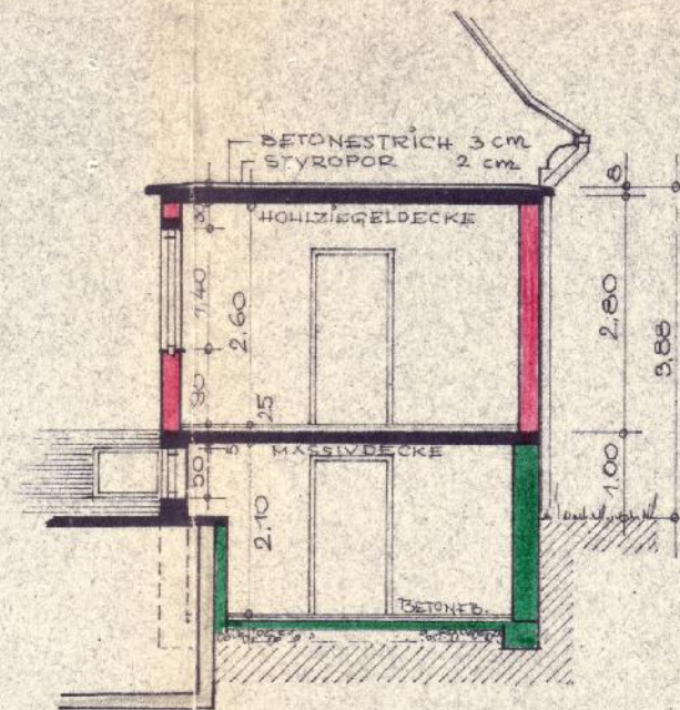
SCHNITT 1-1.
