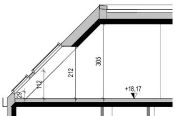
Schnitt 33.C
