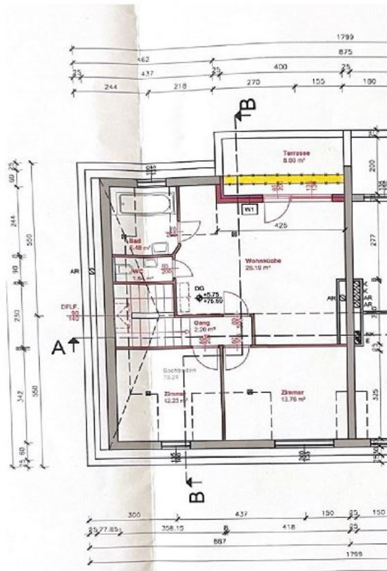
ENTWURF DACHGESCHOSSGRUNDRISS
