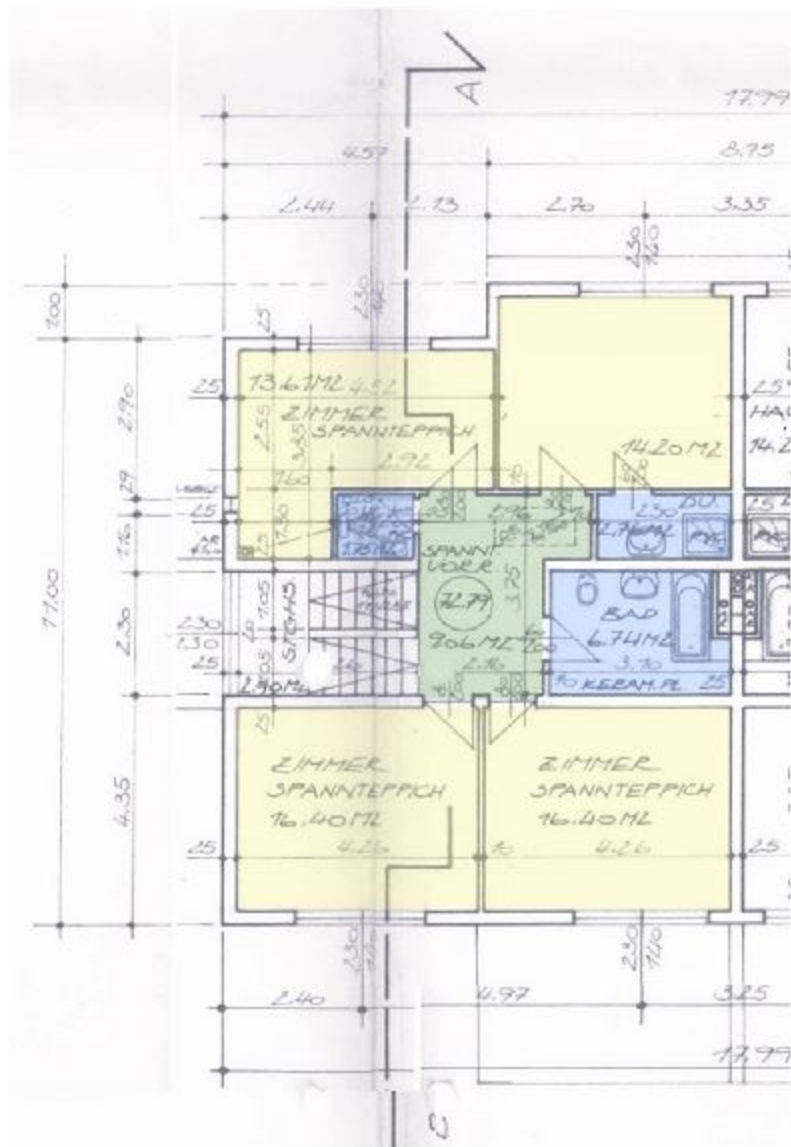
OBERGESCHOSSGRUNDRISS
