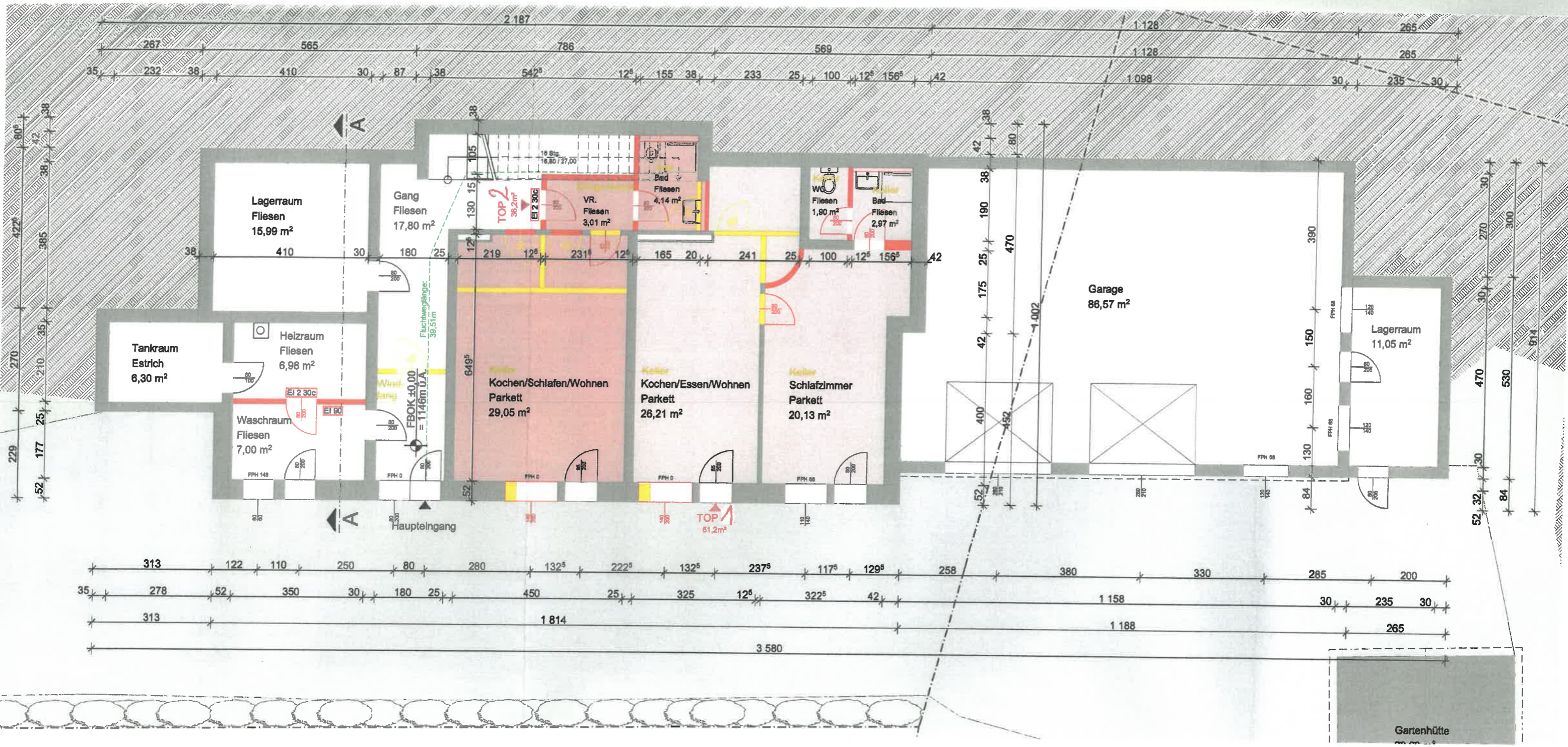
Kellergeschoss 1:
