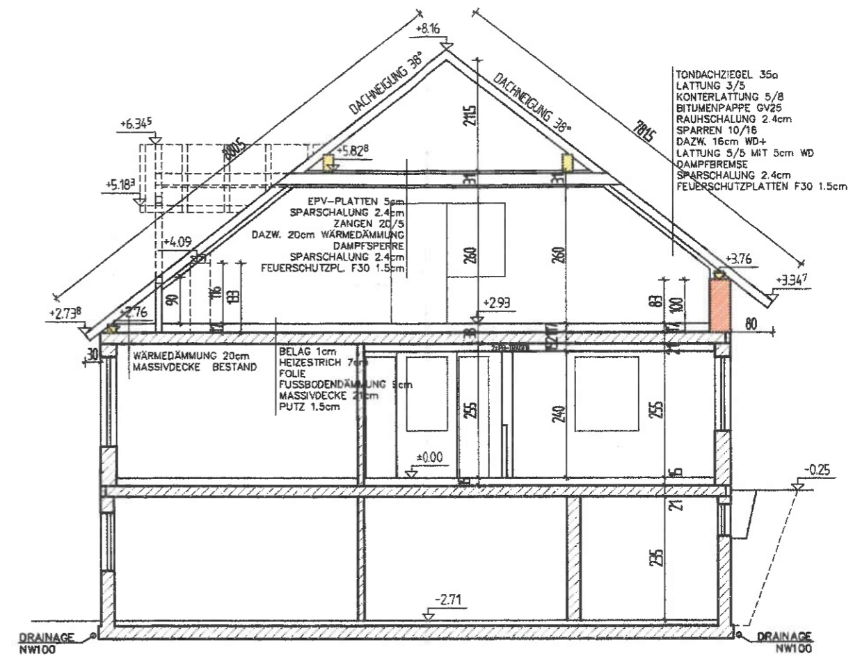
SCHNITT A-A
