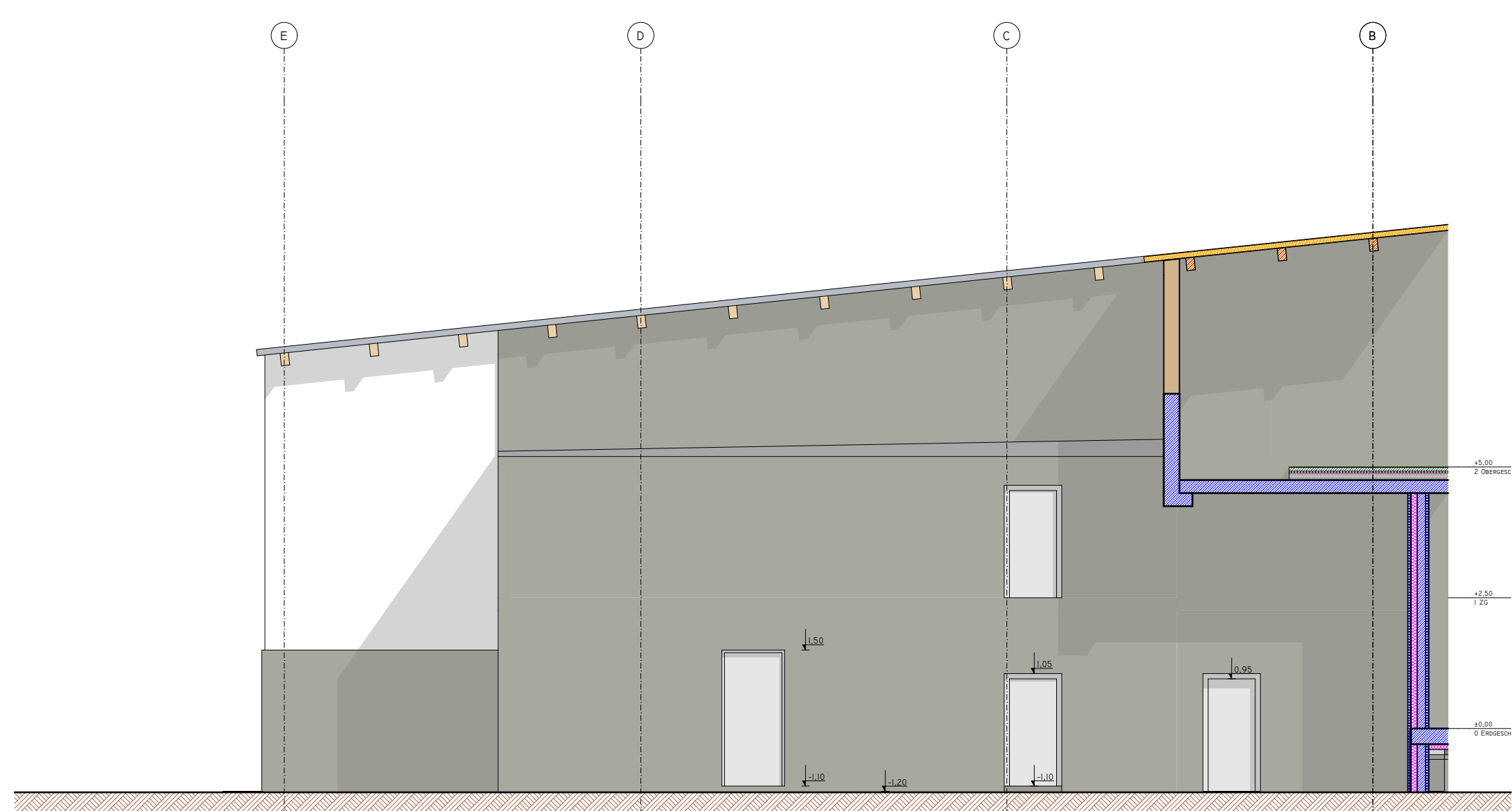
OSTANSICHT (INNENHOF)
