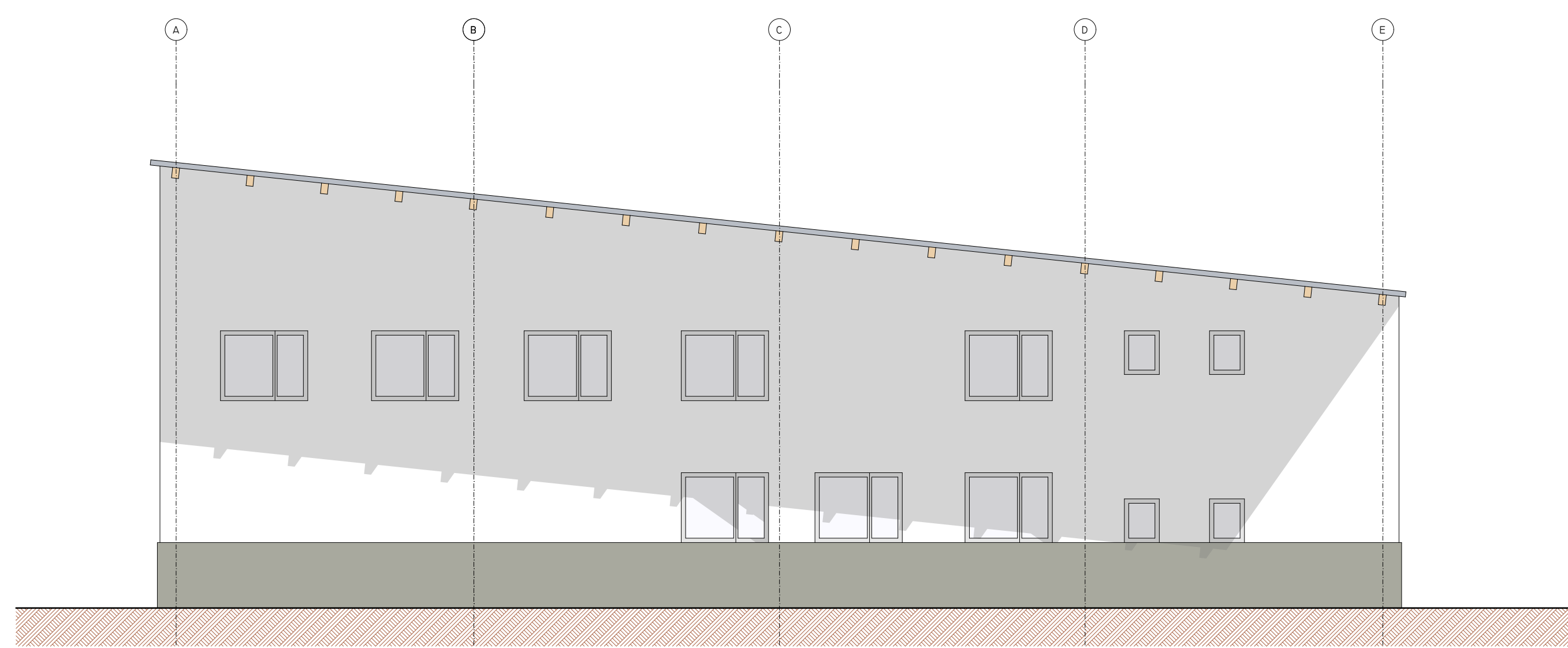
WESTANSICHT
