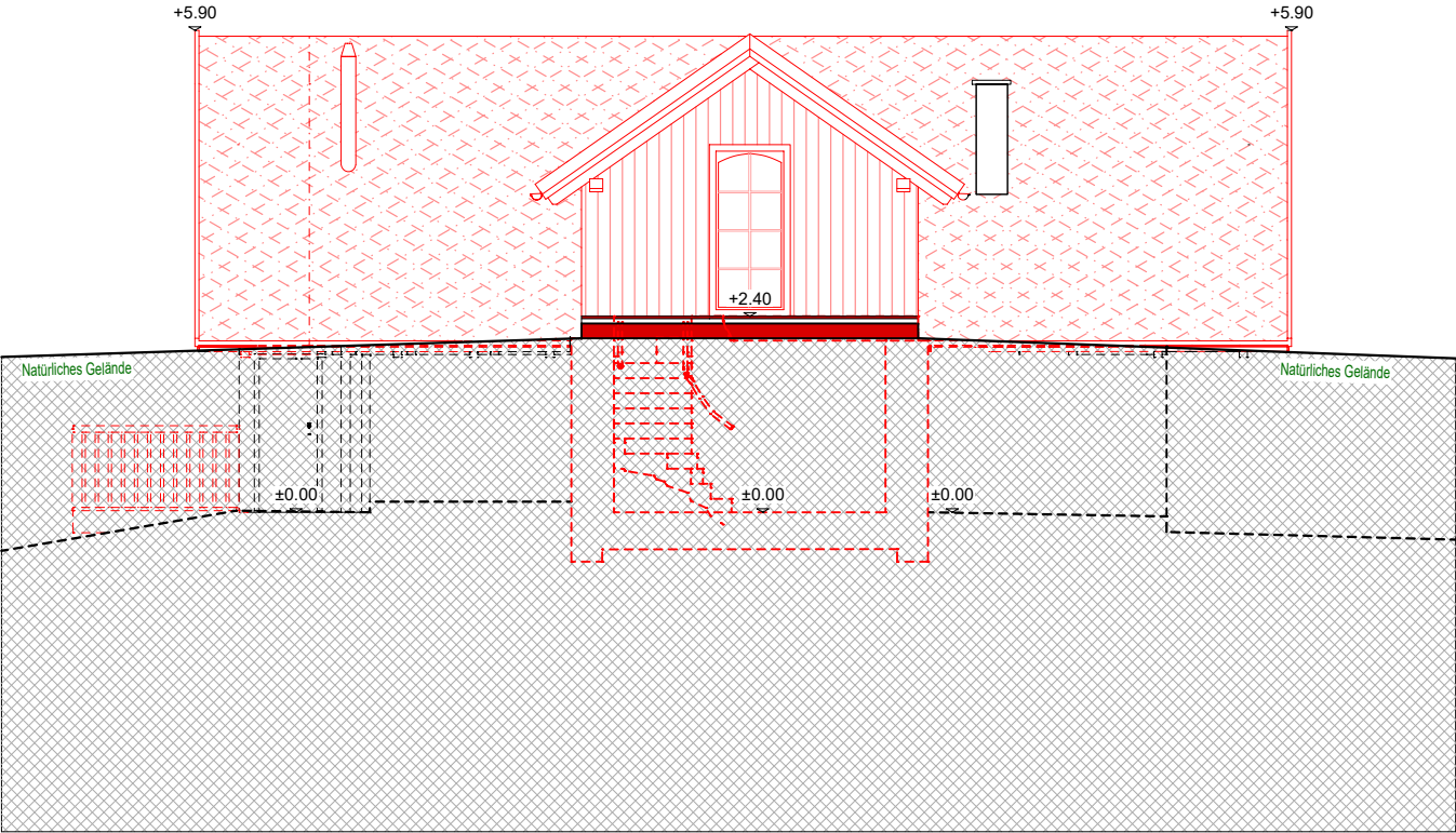
NORDANSICHT
