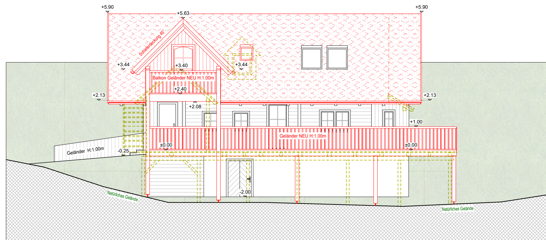
SÜDANSICHT
