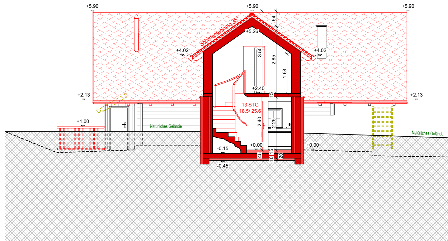
SCHNITT A-A
