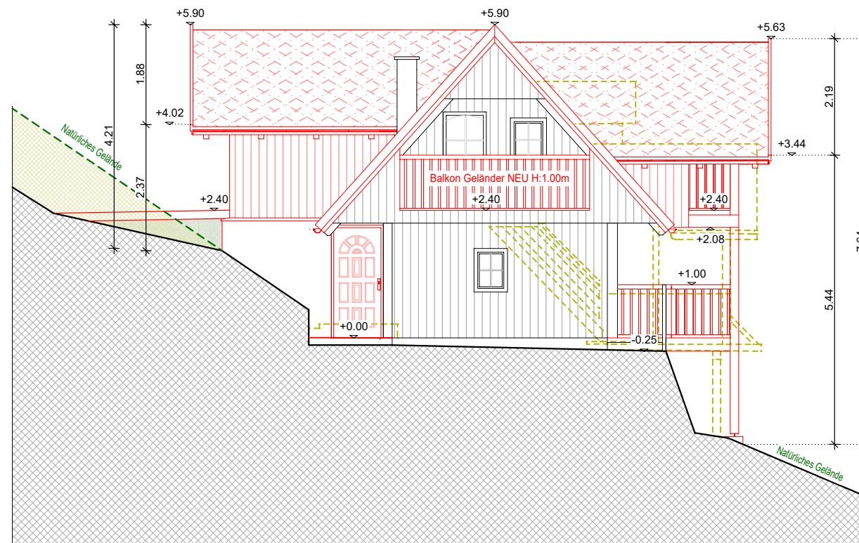
WESTANSICHT
