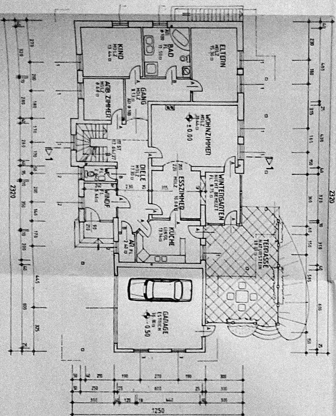
ERDGESCHOSS
