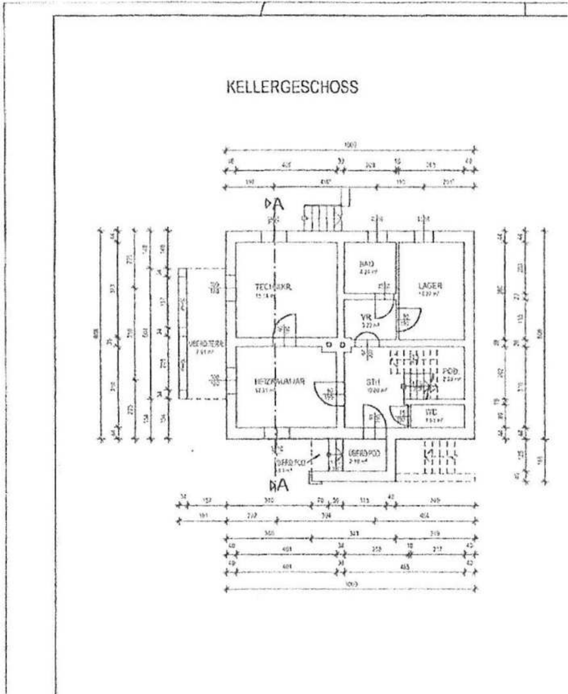
Grundriss KG
