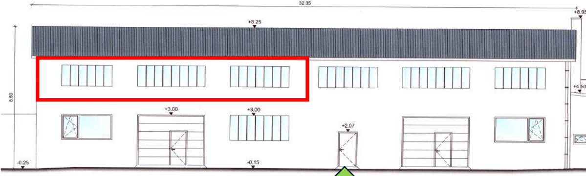
ANSICHT NORD M 1:100
