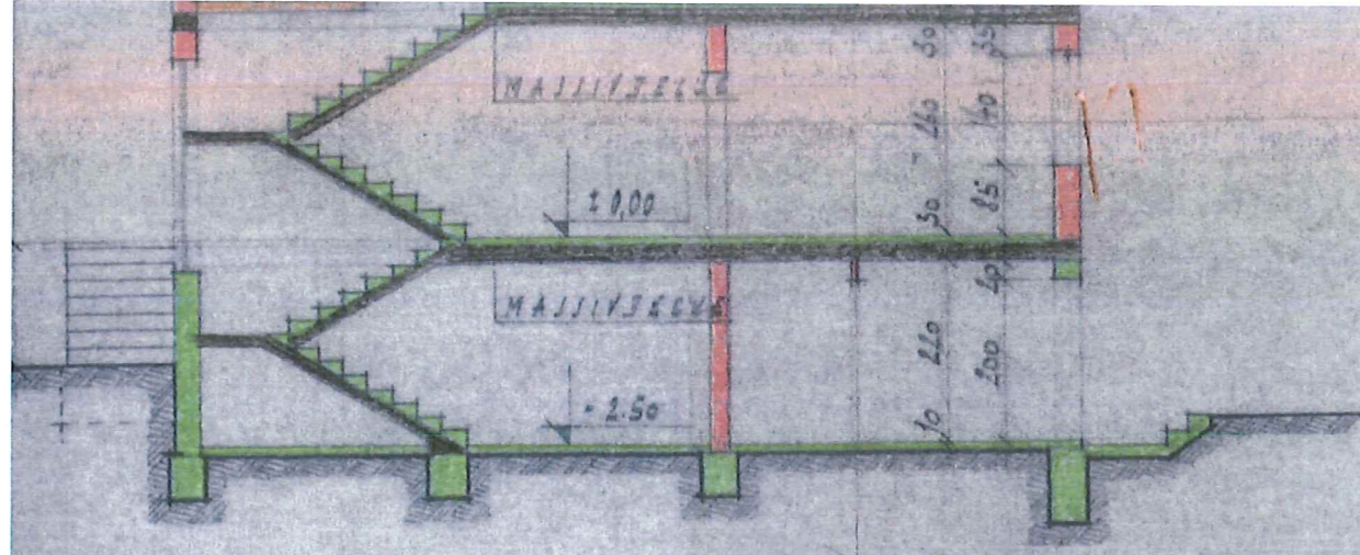
SCHNITT: 1-1
