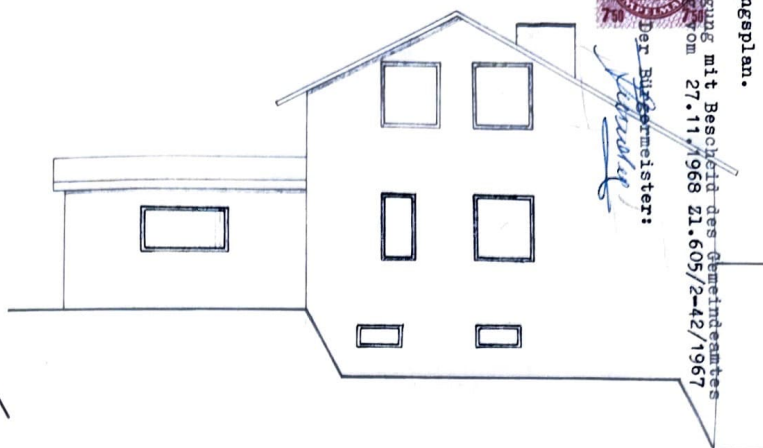
WESTANSICHT
