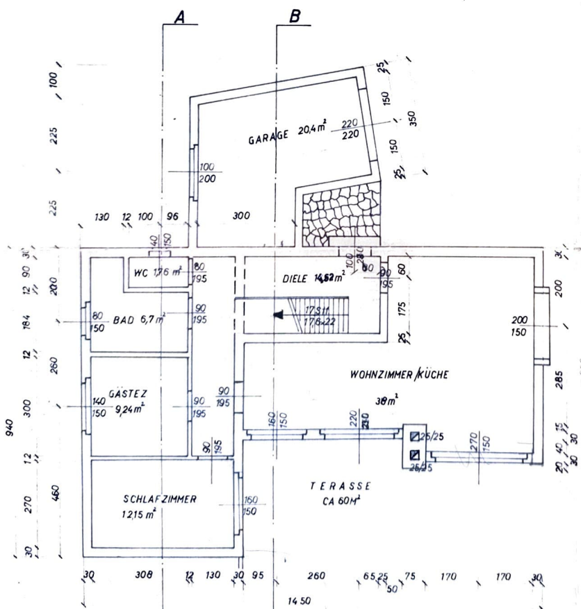
ERDGESCHOSS
