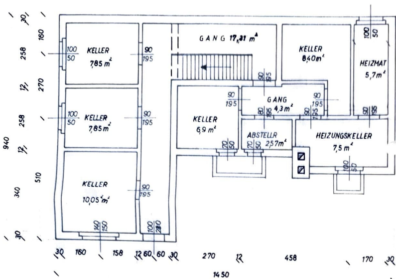
KELLERGESCHOSS
