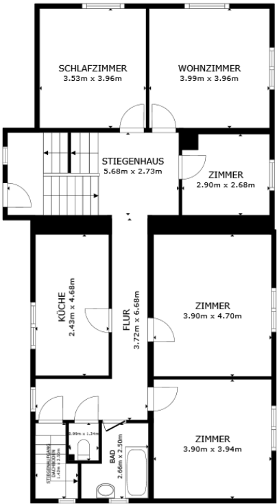
Erdgeschoß
