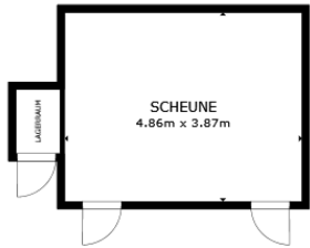
Lagerfläche
