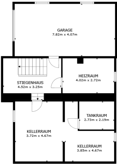
Keller
