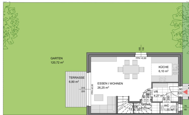
Erdgeschoss
