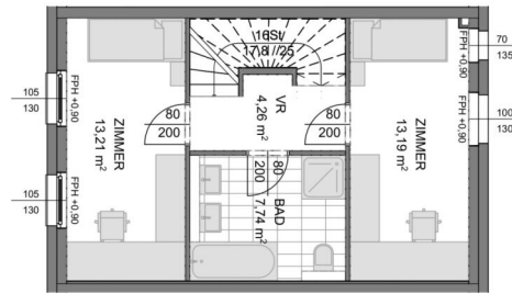
Obergeschoss
