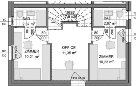
Obergeschoss
