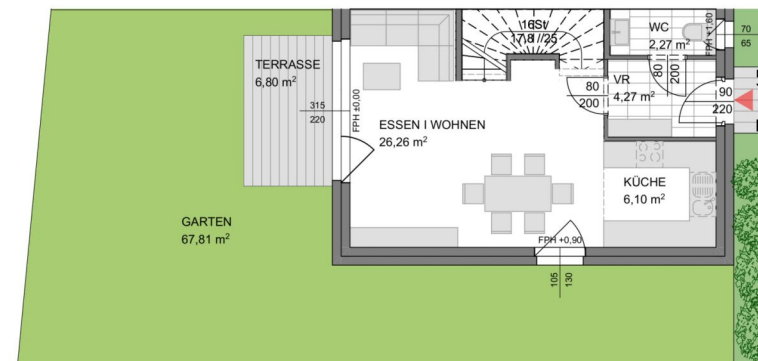
Erdgeschoss
