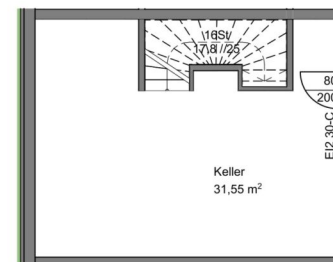
Kellergeschoß
