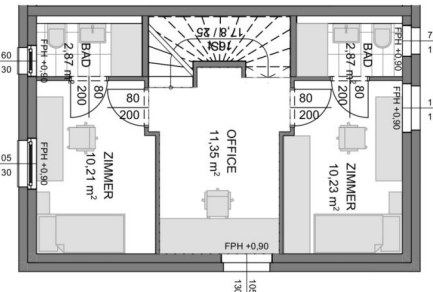
Obergeschoß
