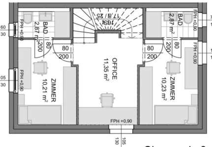
Obergeschoß
