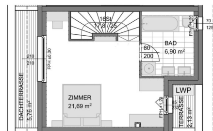
Dachgeschoss
