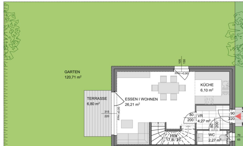
Erdgeschoss
