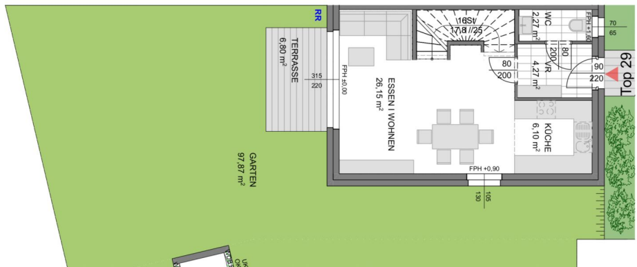
Erdgeschoss
