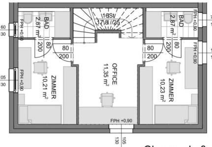
Obergeschoss
