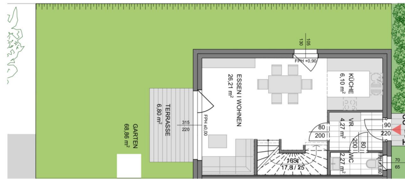
Erdgeschoss
