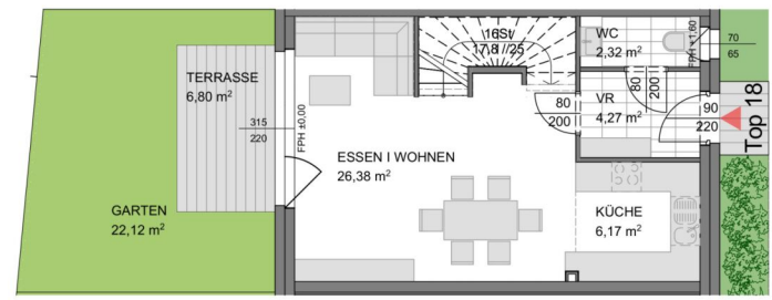
Erdgeschoss
