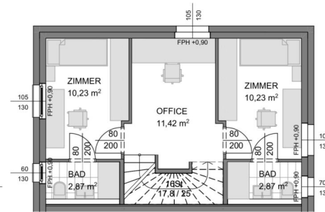
Obergeschöß
