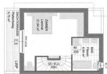
Dachgeschoss
