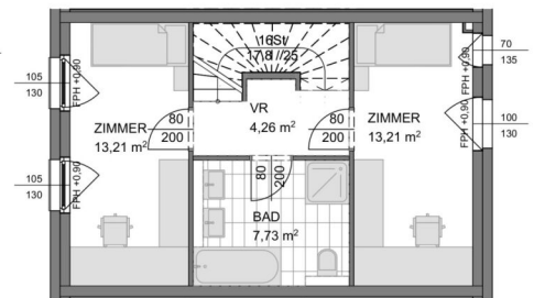
Obergeschoß
