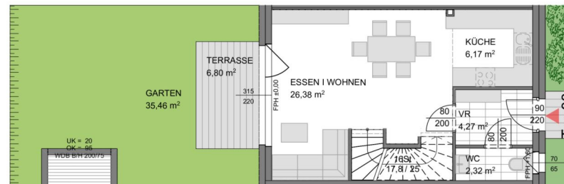
Erdgeschoß
