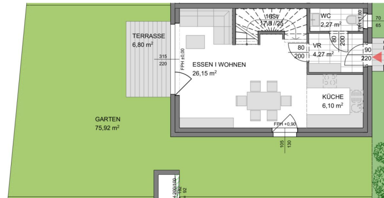
Erdgeschoss
