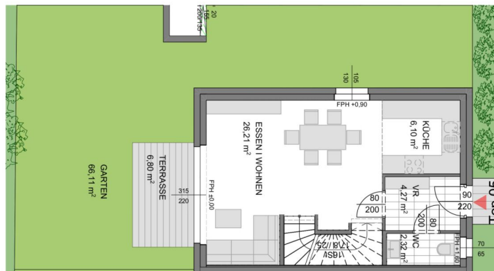
Erdgeschoss
