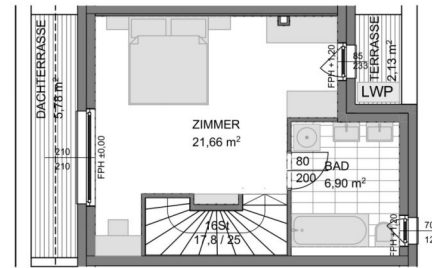
Dachgeschoß
