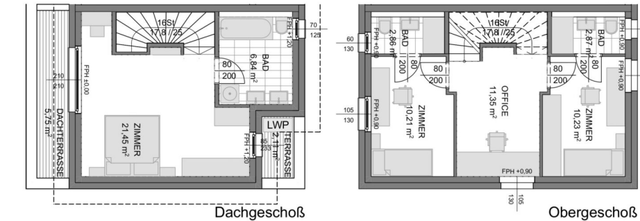
Dachgeschoss
