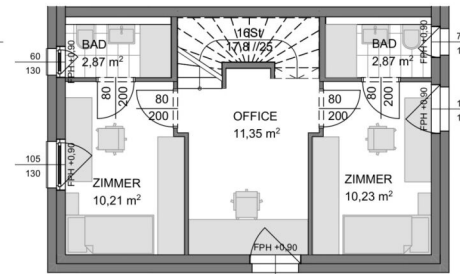
Obergeschoss
