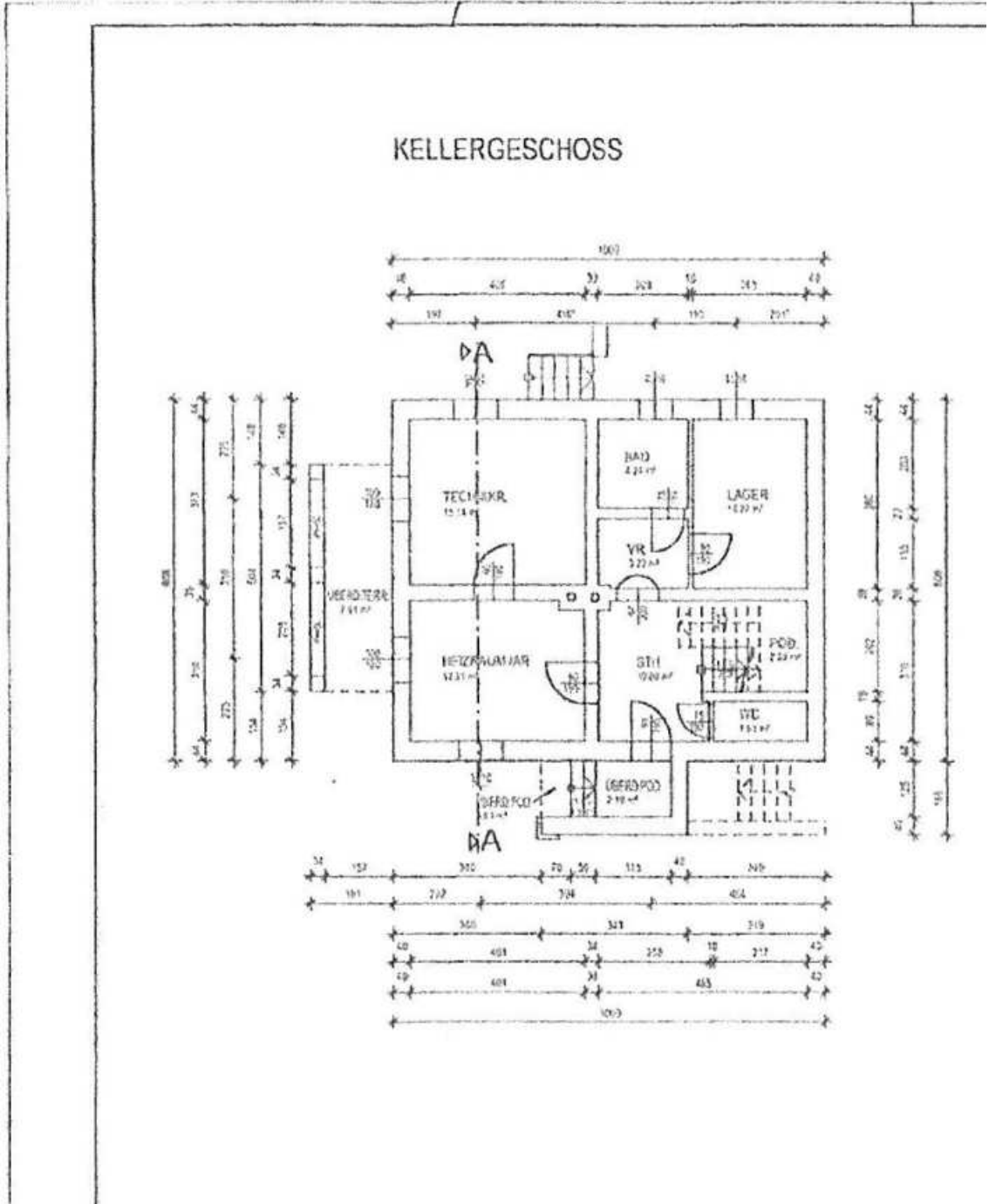
Grundriss KG
