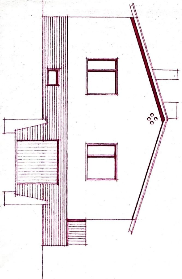
WESTANSICHT
