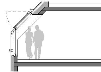
SCHNITT A
