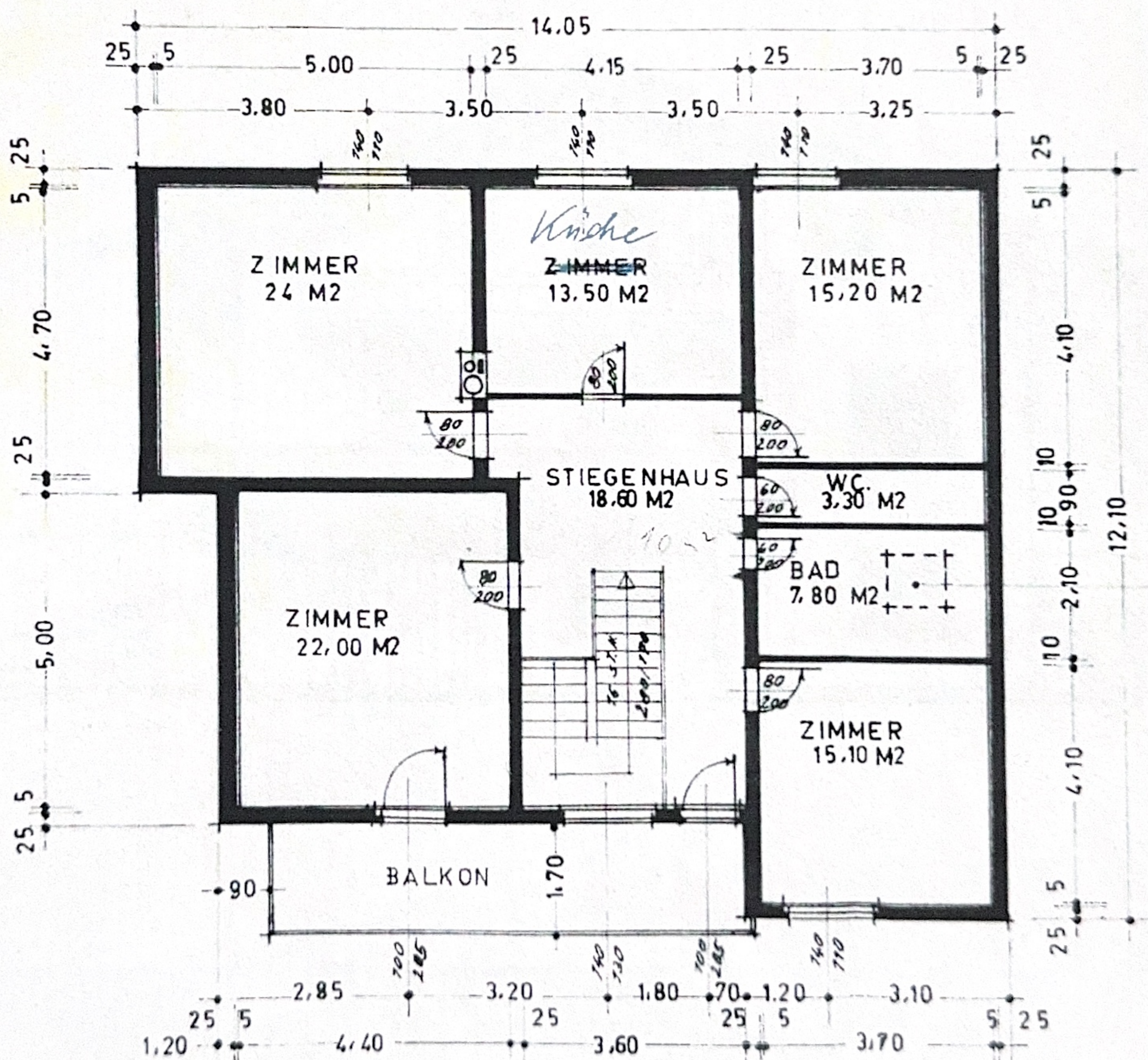
DACHGESCHOSS GRUNDRISS
