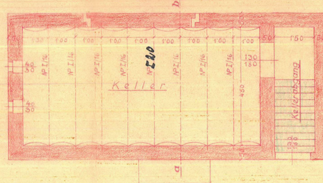
Keller - Grundriss
