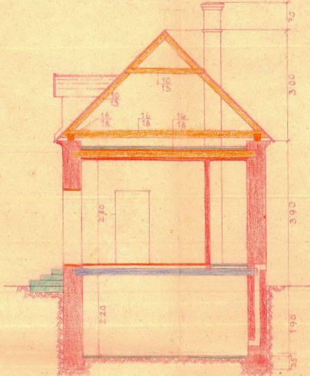
Schnitt a-b
