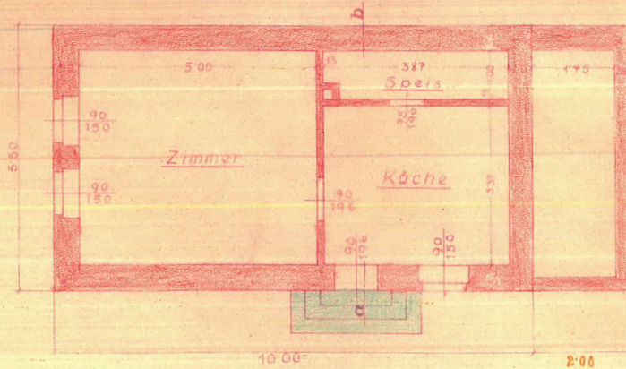
Erdgeschoss - Grundriss
