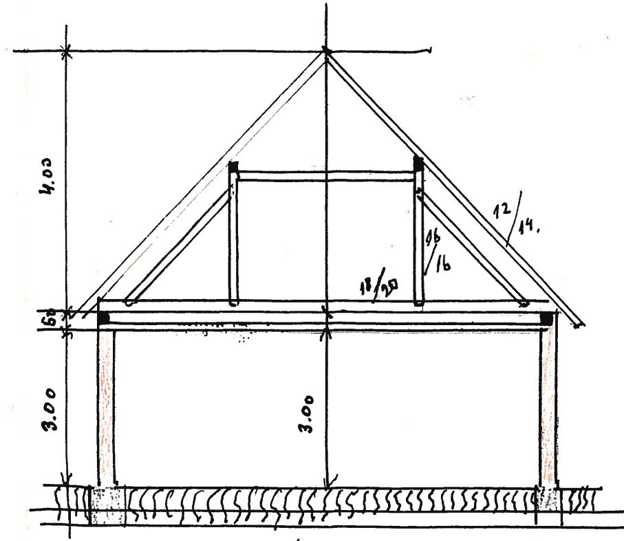
Schnitt a-b
