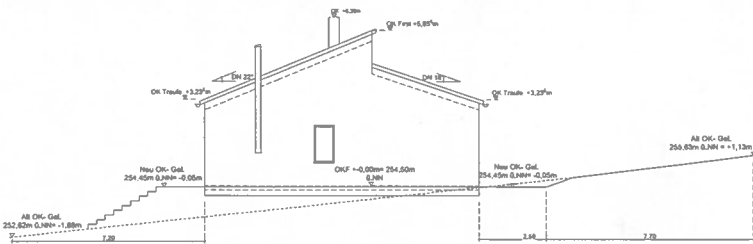
Nordwest Ansicht M 1 : 100
