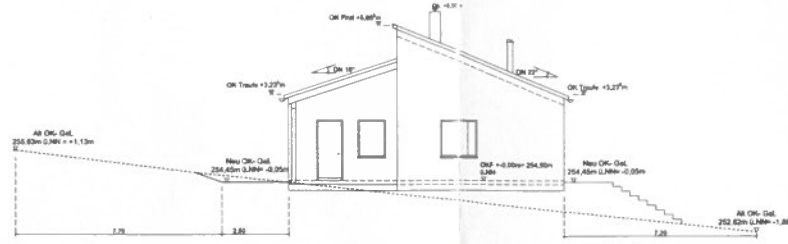
Südost Ansicht M 1 : 100
