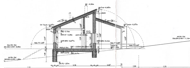
Schnitt A M 1 : 100
