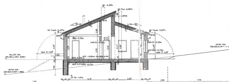
Schnitt B M 1 : 100
