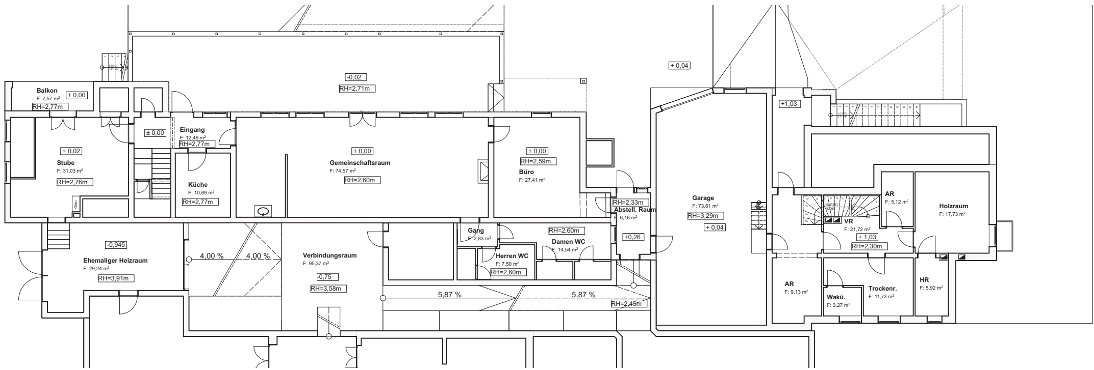
Erdgeschoss Wohnbereich
