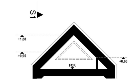
Schnitt 2
