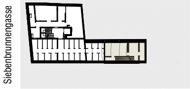
Grundriss Untergeschoss
