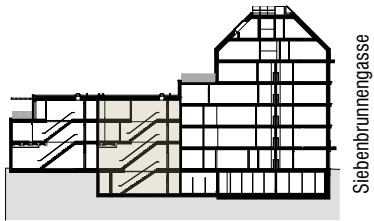
Schnitt
