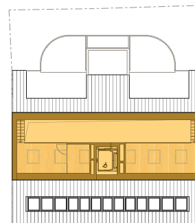
DG Empore
